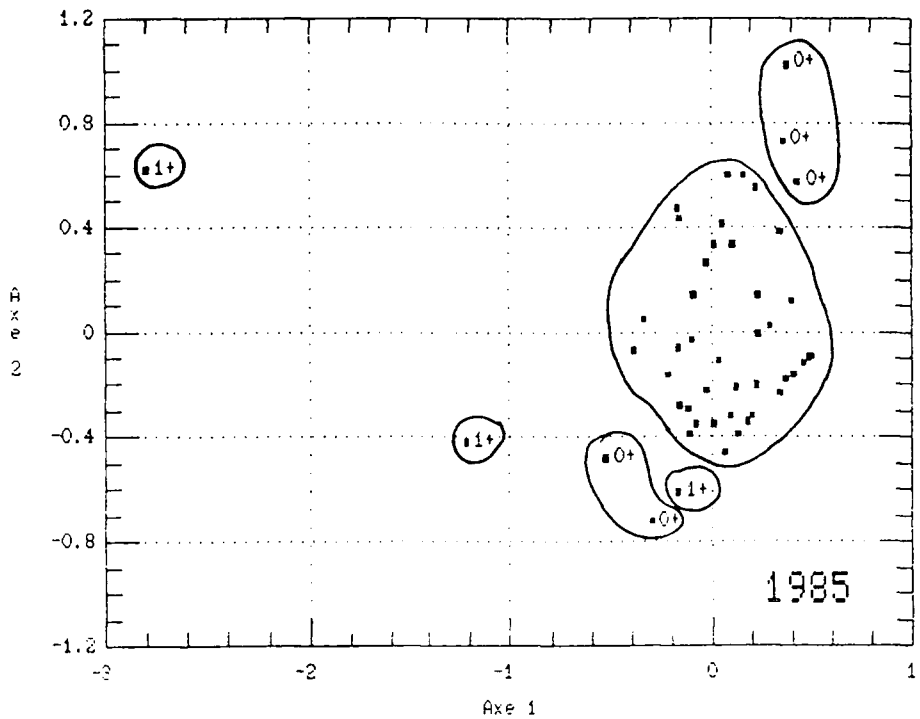
figure 4 : Ordination des truites du cycle de 1985 selon les deux premiers axes déterminés par l'analyse en composantes principales. Variabilité sur les deux axes : 41,7 % ; corrélation avec données originales : 93,4 %.
