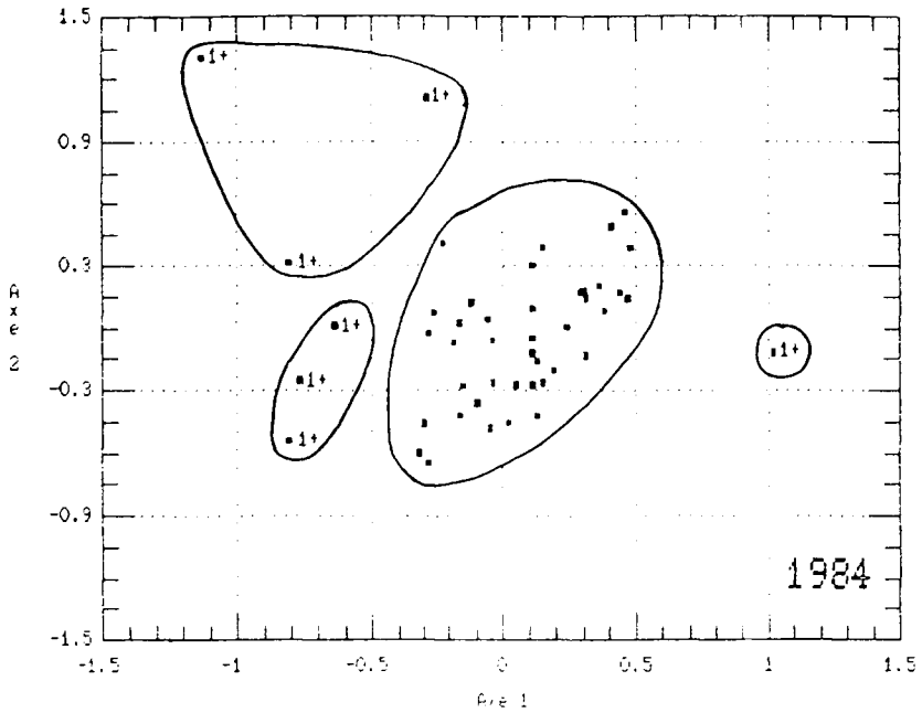
figure 3 : Ordination des truites du cycle de 1984 selon les deux premiers axes déterminés par l'analyse en composantes principales. Variabilité sur les deux axes : 30,8 % ; corrélations avec données originales : 80,8 %.
