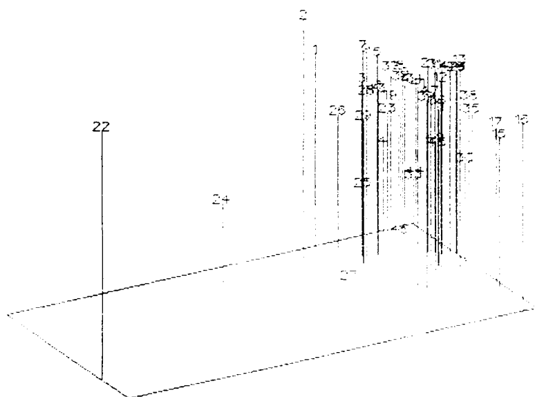
figure 5 : Ordination des truites du cycle de 1985 selon les trois premiers axes déterminés par l'analyse en composantes principales. Variabilité sur les trois axes : 54,6 % ; corrélation avec données originales : 93,4 %.
