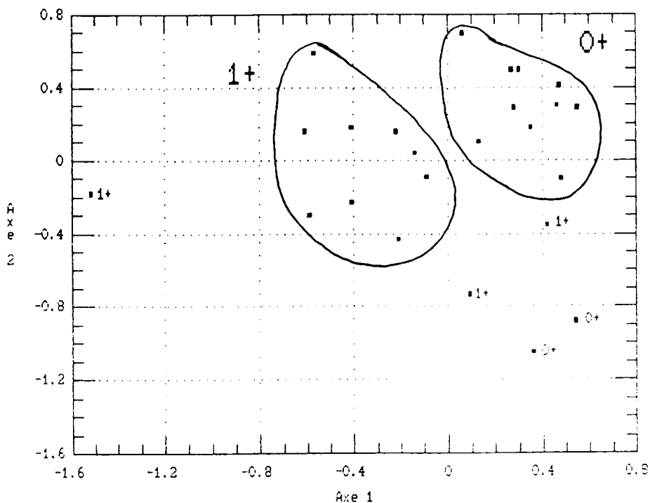
figure 6 : Ordination des truites, regroupées selon l'heure de récolte, pour les deux cycles d'alimentation. Variabilité sur les deux axes : 45,5 % ; corrélation avec données originales : 90,4 %.
